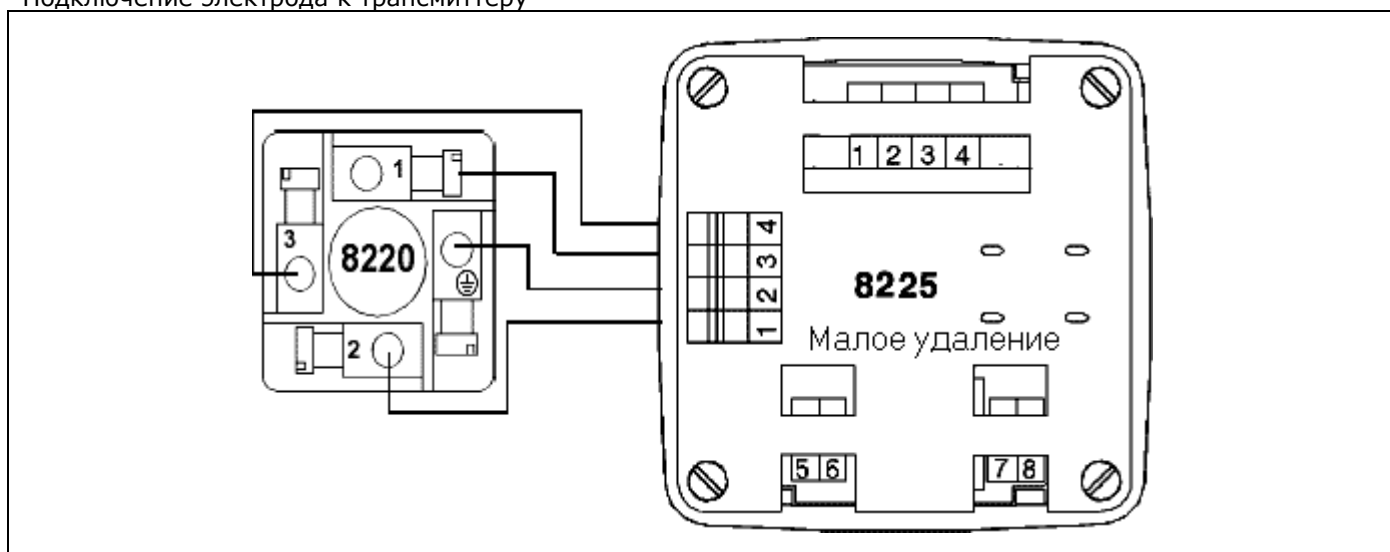
Рис. 3.10 Трансмиситтер 8225 с реле, малое удаление
