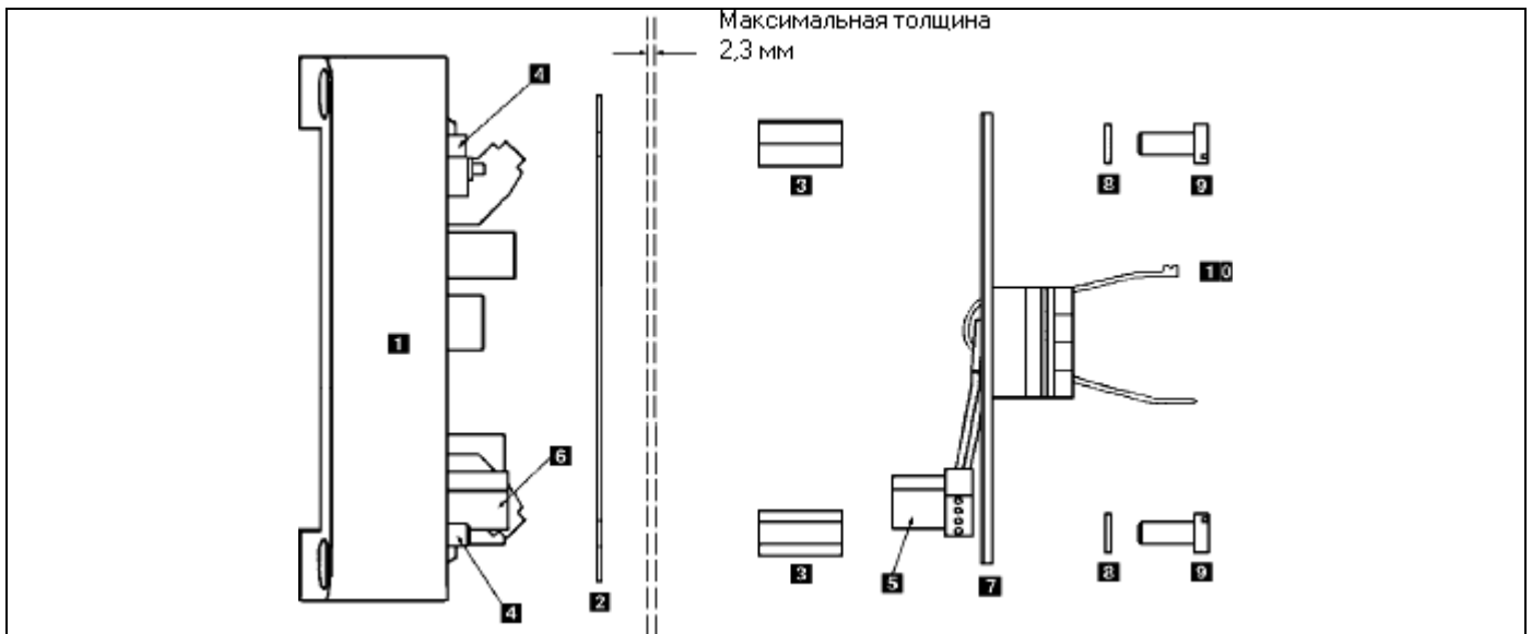
Рис. 3.2 Установка трансмиттера 8225, панельное исполнение
